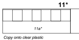
PL01 - Tater Du
