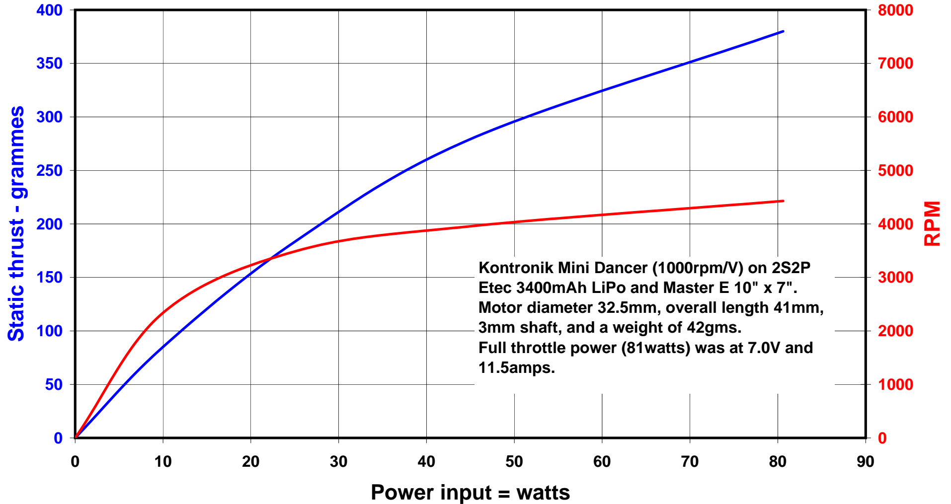
Graph 7 - Kontronik Mini Dancer.
